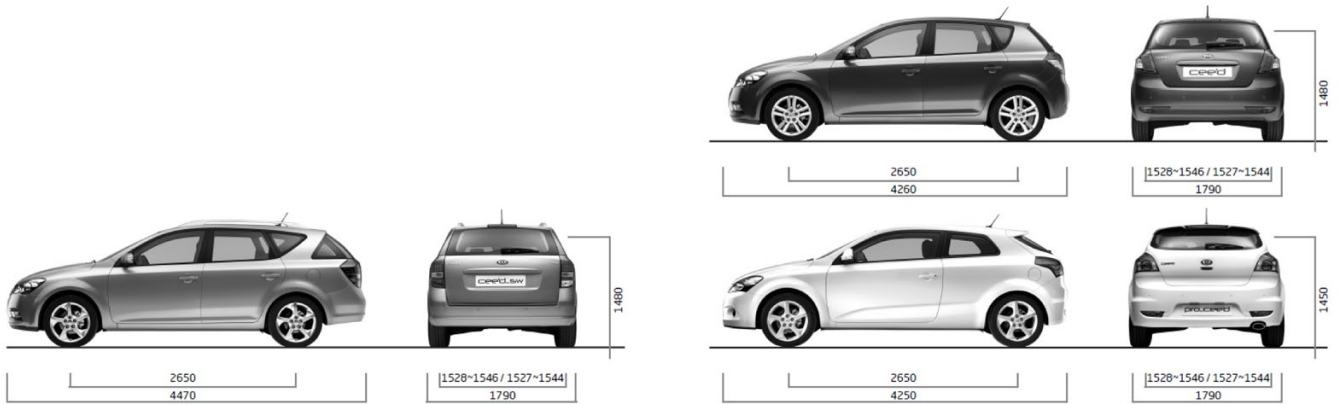
Wymiary [mm]
